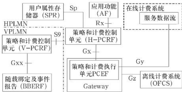
图1 PCC标准架构示意图(用户漫游使用归属地网络)
