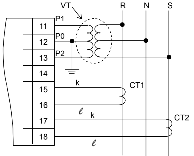
单相 3 线式的接线
