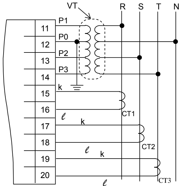
三相 4 线式的接线
