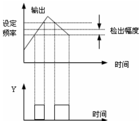
图 4-26 频率到达信号输出示意图
