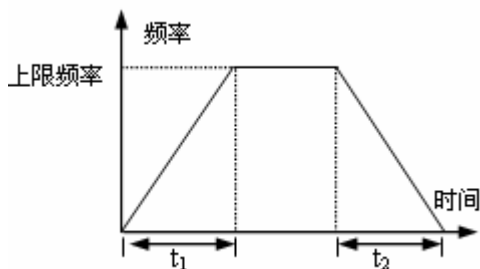
图 4-4 直线加减速
