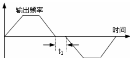
图 4-1 正反转死区时间
