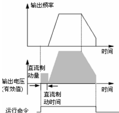
图 4-11 起动方式 1 说明
