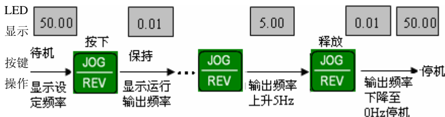
图 3-9 点动运行操作示例
