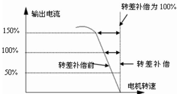
图 4-13 转差频率补偿示意图
