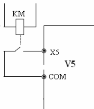
图 4-20 外部设备故障输入示意图
