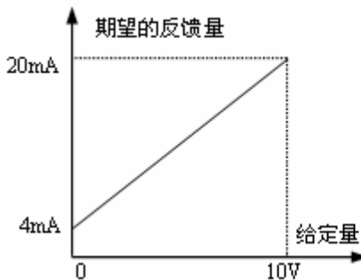
图 4-34 给定量和期望反馈量
