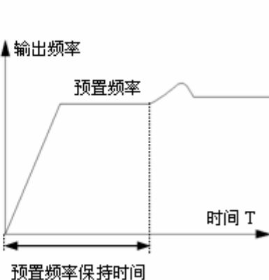
图 4-38 闭环预置频率运行示意图
