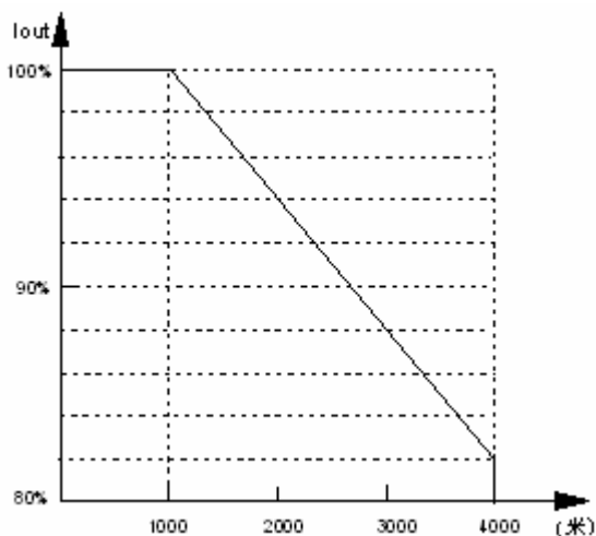
图 0-2 变频器额定输出电流与海拔高度降额使用图
