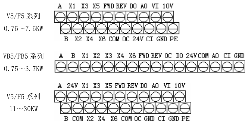
图 2-5 控制板端子排列顺序图
