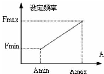
(1)正作用特性
