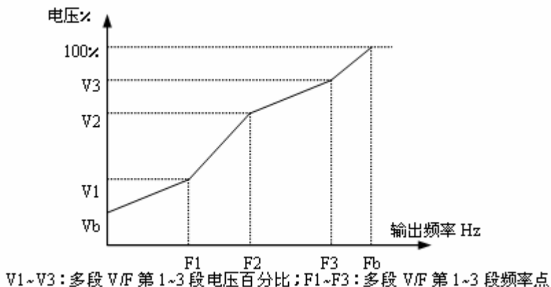
图 4—8 用户定义 V/F 曲线
