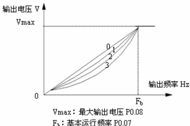
图 4—7 V/F 曲线
