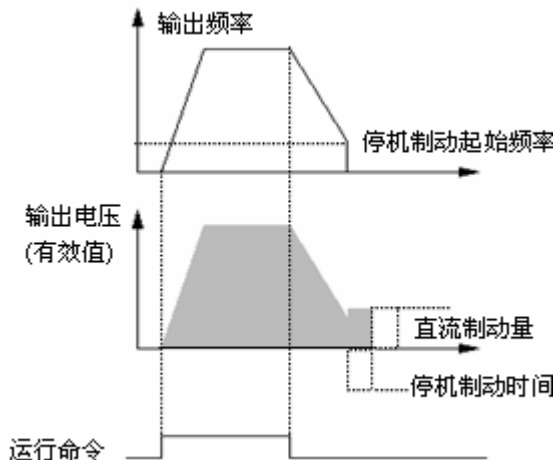
图 4-12 减速停车+直流制动示意图
