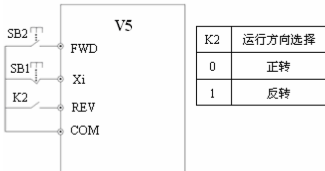
图 6-24 三线式运转模式 2
