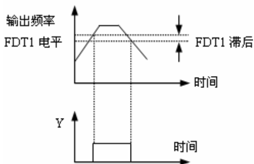
图 4-27 频率水平检测示意图
