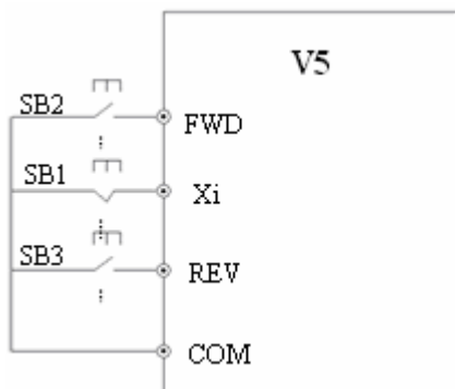
图 4-23 三线式运转模式 1
