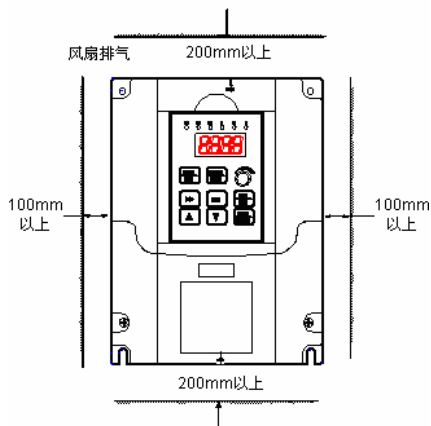
图 2-1 安装的间隔距离图
