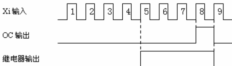
图 4—28 设定计数值给定和中间计数值给定示意图
