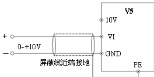
图 2-6 VI 端子配线图
