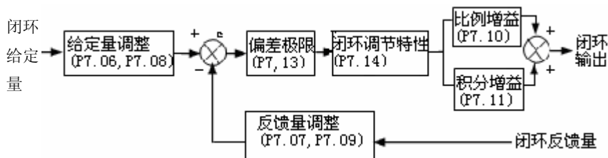
图 4-33 PI 控制原理框图
