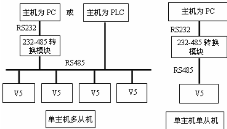
图 7-1 从机组网方式示意图
