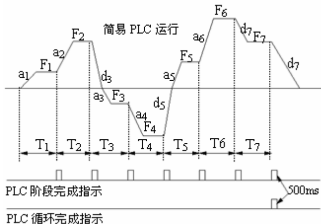
图 4-40 简易 PLC 运行图
