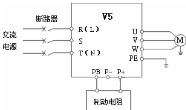
图 2-3 主回路简单配线
