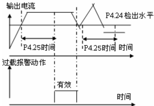
图 4-29 过载报警
