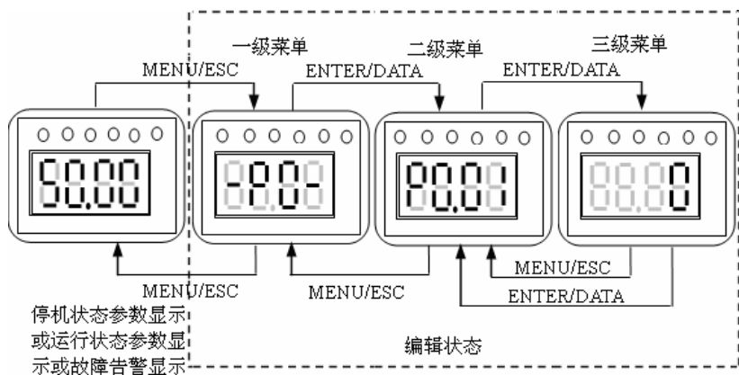
图 3-6 操作面板编程显示状态
