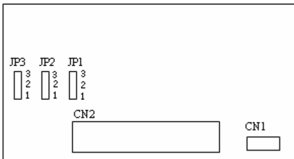
图 2-4 (c) 控制板端子跳线位置示意图
