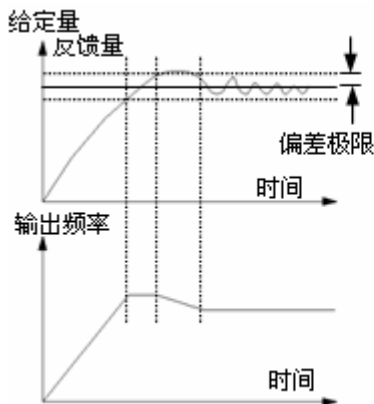
图 4-37 偏差极限示意图
