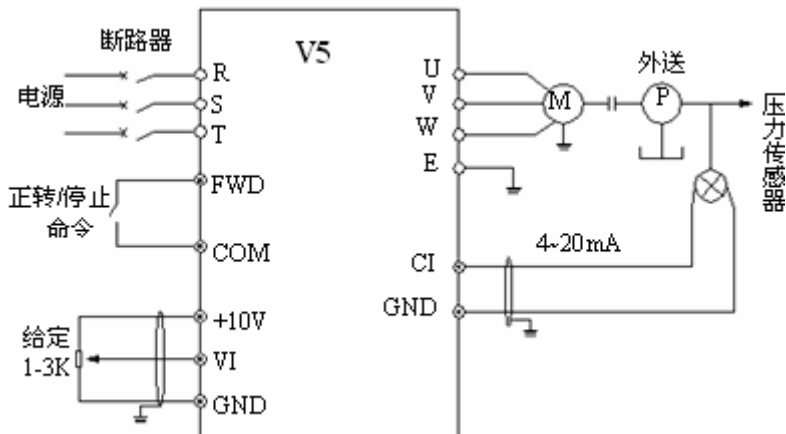
图 4-32 内置 PI 模拟反馈控制系统示意图
