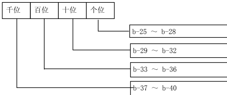
图 4-17 显示参数选择 2 示意图
