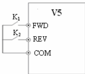
图 4-21 两线式运转模式 1
