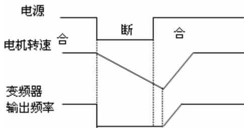
图 4-9 转速跟踪再启动示意图
