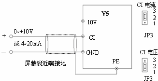
图 2-7 CI 端子配线图
