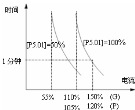
图 4-30 电子热继电器保护
