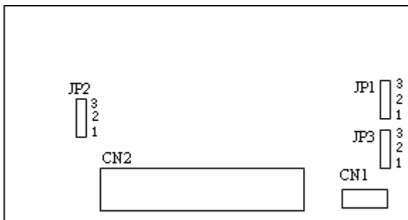
图 2-4 (a) 控制板端子跳线位置示意图
