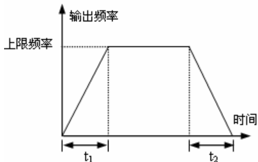
图 4-6 加减速时间定义
