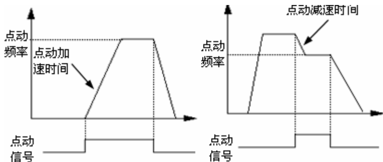
图 4-14 点动运行
