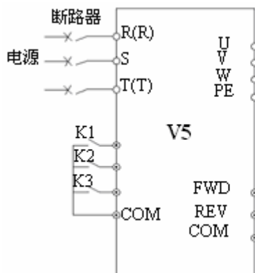
图 4-19 多段速运行接线图
