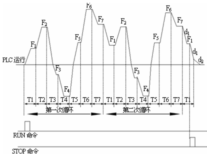
图 4-43 PLC 连续循环方式
