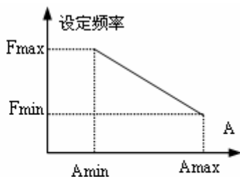
(2)反作用特性
