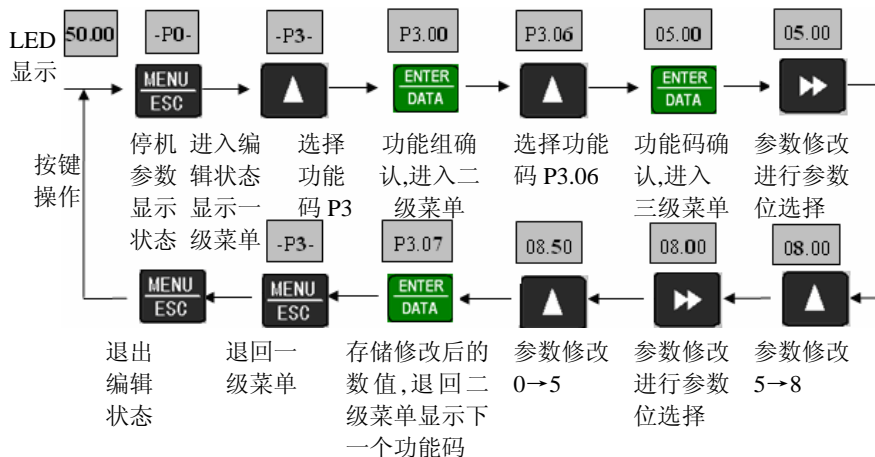
图 3-8 参数编辑操作示例
