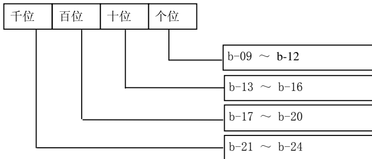
图 4-16 显示参数选择 1 示意图
