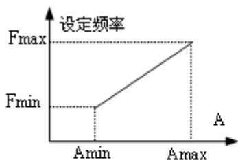
(1)正作用特性
