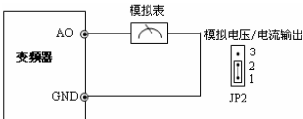
图 2-8 模拟输出端子配线
