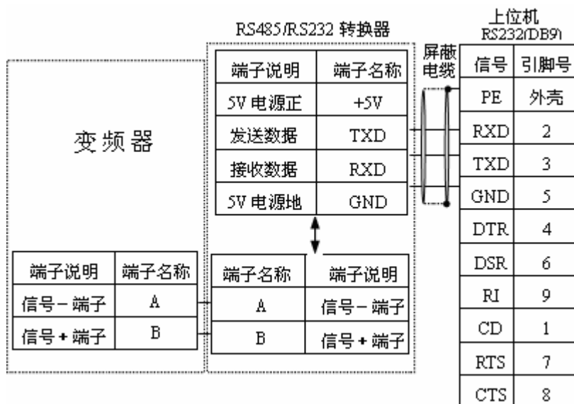
图 2-9 RS485—(RS485/232)—RS232 通讯配线
