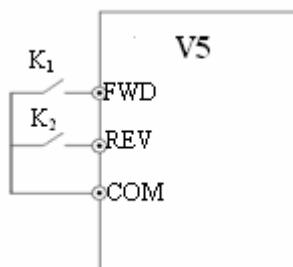
图 4-22 两线式运转模式 2
