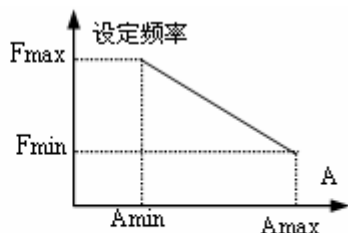
(2)反作用特性
