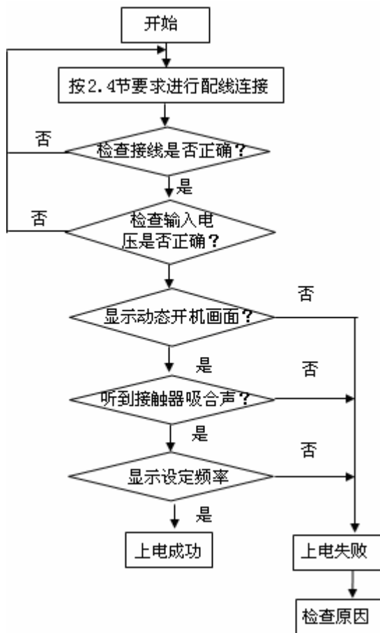
图 3-12 变频器初次上电操作流程
