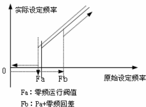
图 4-39 零频回差运行
