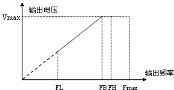
图 4-2 特性参数定义示意图
