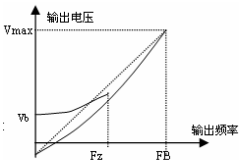
(a) 恒转矩曲线转矩提升示意图
