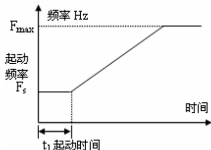
图 4-10 起动频率与起动时间示意图
