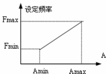
(1)正作用特性
