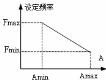
(2)反作用特性
