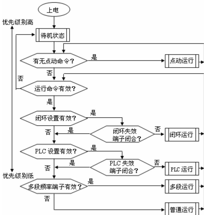
图 3-1 变频器运行状态的逻辑关系图
