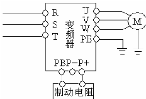
图 1-1 变频器与制动组件连线图
