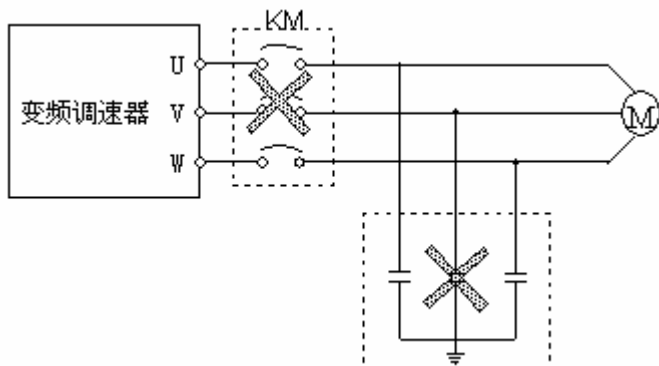
图 0-1 变频器输出端禁止使用电容器
