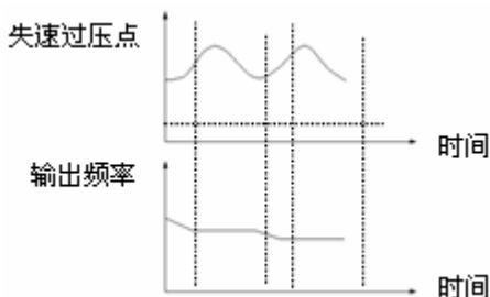
图 4-31 过压失速功能
