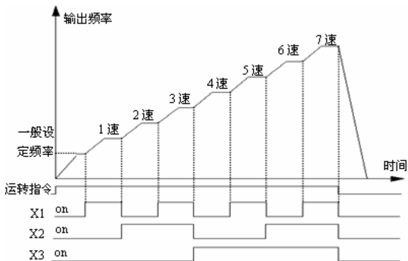
图 4-18 多段速运行示意图
