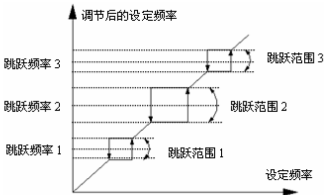
图 4-15 跳跃频率及范围示意图
