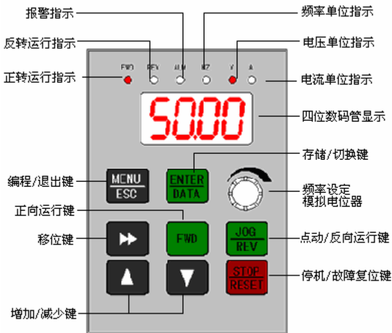
图 3-2 操作面板功能图
