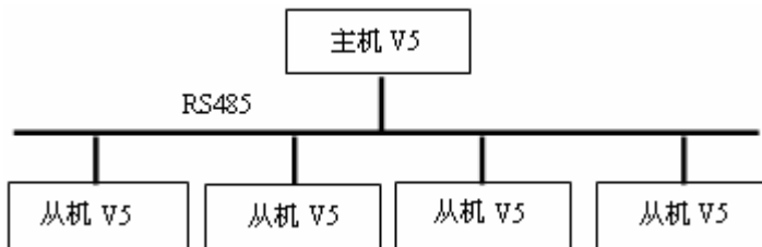
图 7-2 多机联动组网示意图
