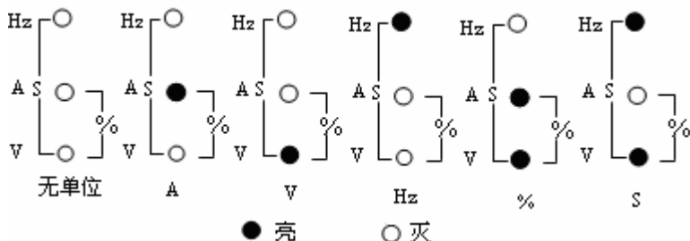
图 3-3 单位指示灯状态与单位关系图
