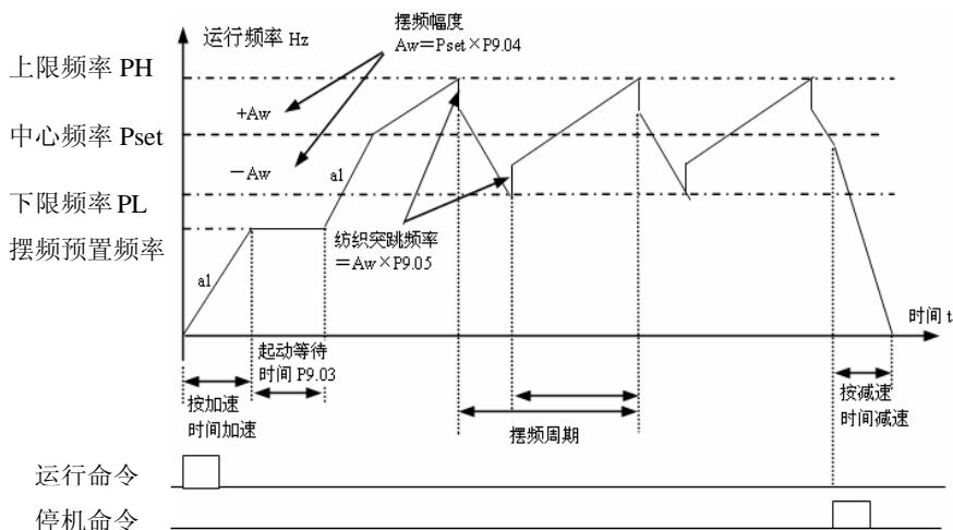
图 4—45 摆频运行示意图
