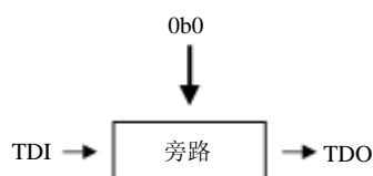
图 12-4 JTAG 旁路寄存器操作
