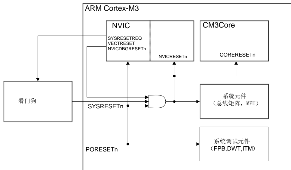
图 6-1 复位信号
