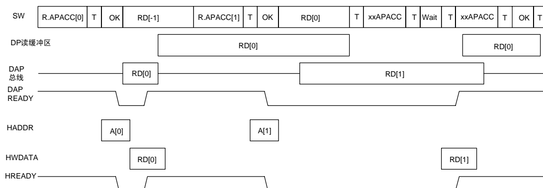
图 12-17 读操作时 SW-DP 到 DAP 总线的时序
