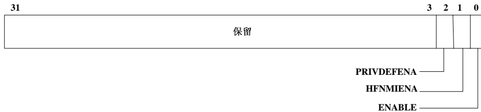
图 9-2 MPU 控制寄存器的位分配
