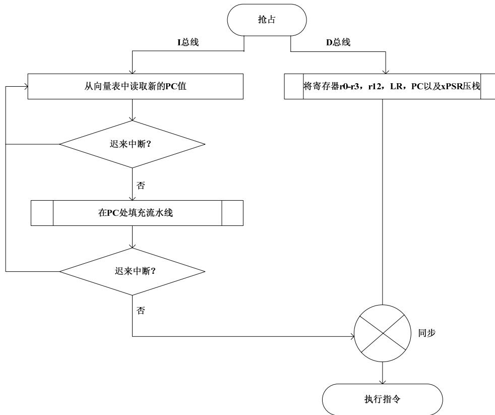
图 5-7 占先流程
