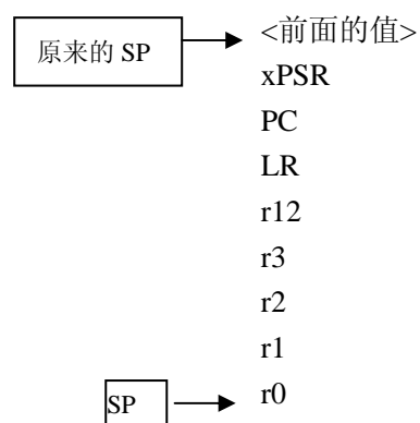
图 5-1 抢占之后堆栈中的内容
