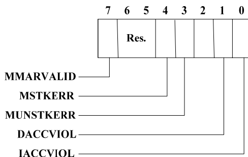
图 8-16 存储器管理故障寄存器的位分配
