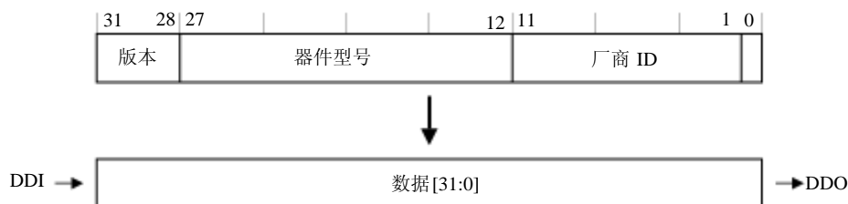
图 12-5 JTAG 设备 ID 代码寄存器位顺序
