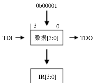
图 12-3 JTAG 指令寄存器位顺序
