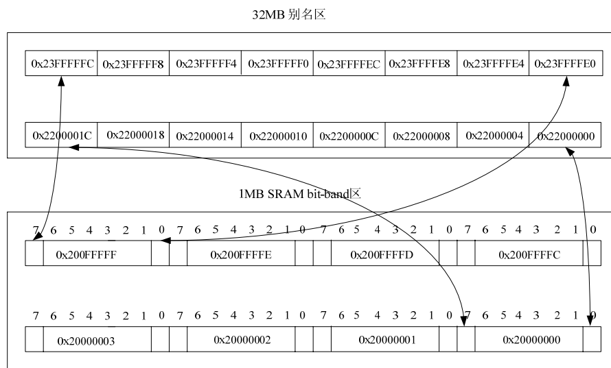
图 4-2 bit-band 映射
