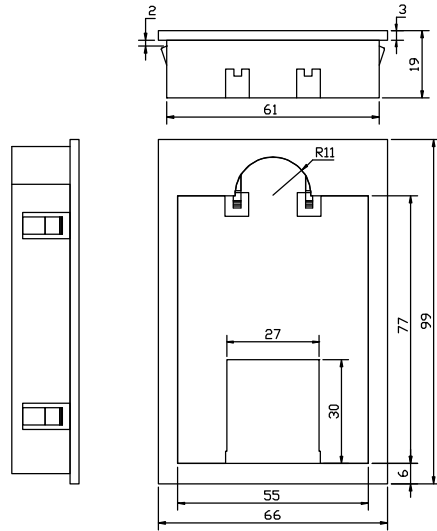
小键盘仓 JP5D7800 尺寸图:
