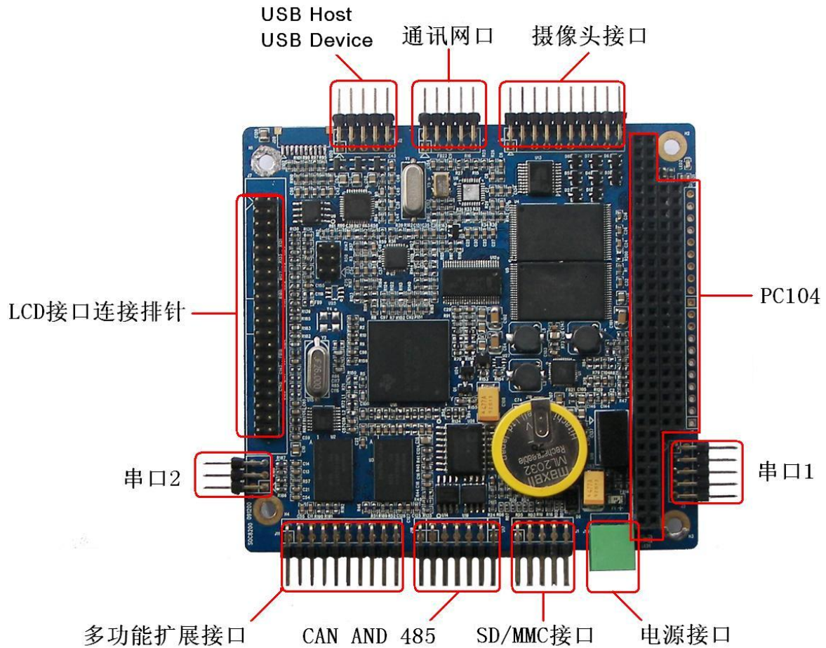
SOC8200 工业单板机接口示意图
