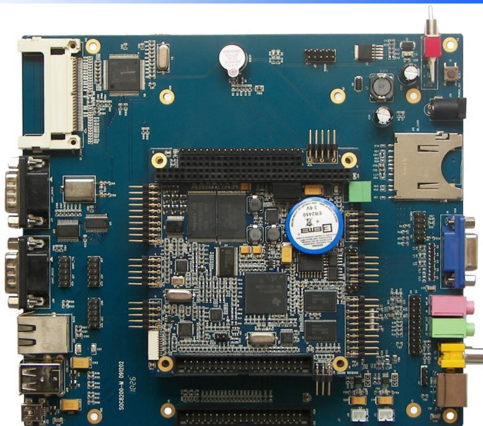
SOC8200 工业单板机 + 扩展底板图
