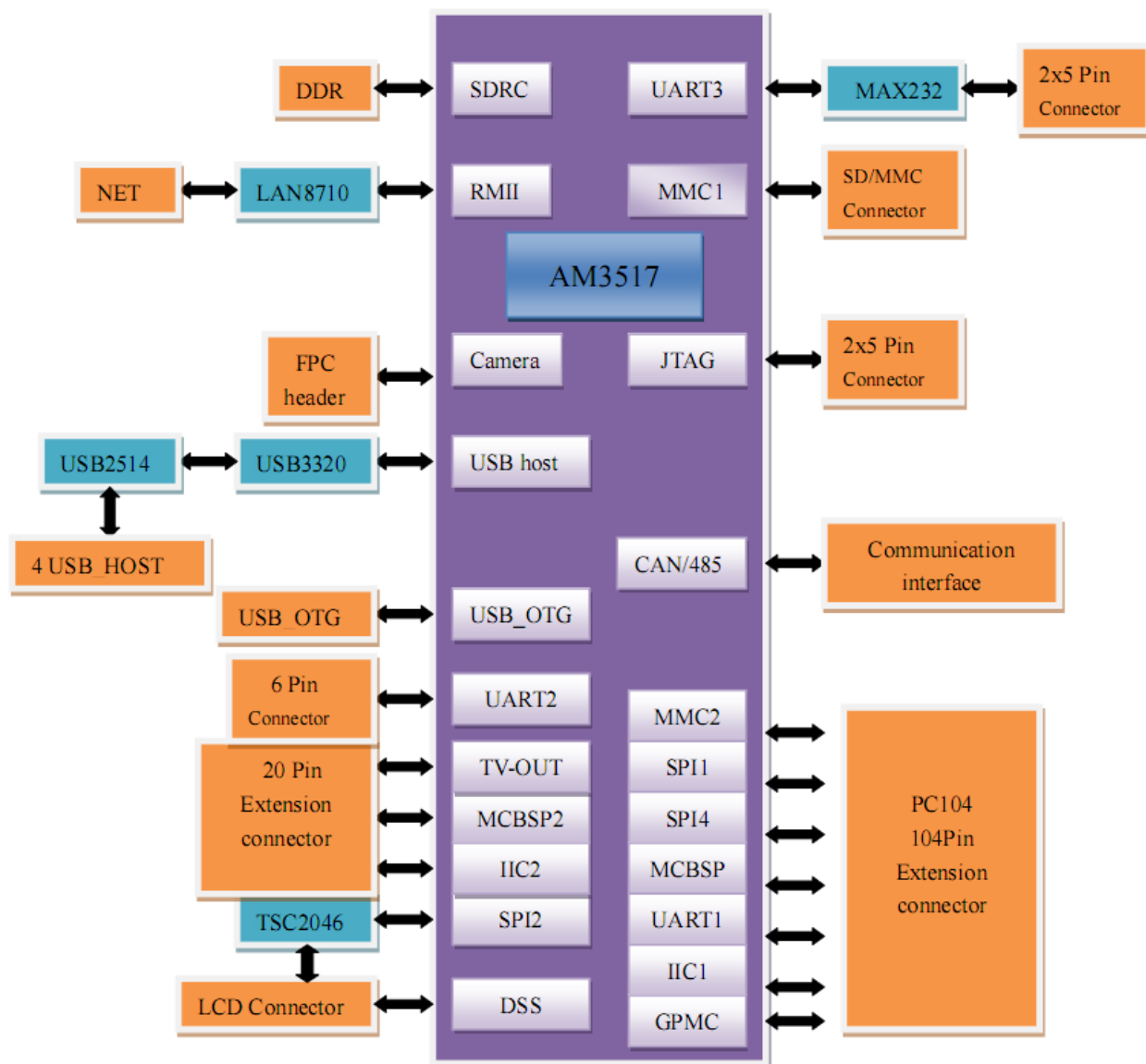
SOC8200 工业单板机系统框图
