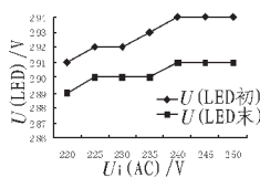
图7 不同输入电压下LED电压变化
