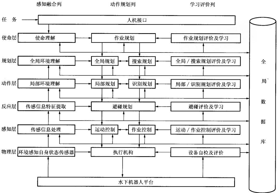
图 4 智能水下机器人软件体系结构图
