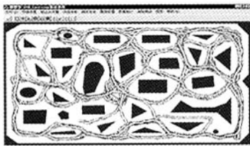
图 7 机器人经过一段时间学习后的运动轨迹
