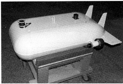
图 2 微小型水下机器人载体“微龙- I 号” Fig. 2 Mini underwater vehicle “WEILONG- I”
