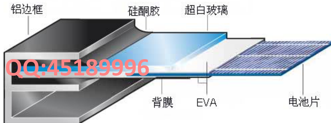
组件结构示意图
