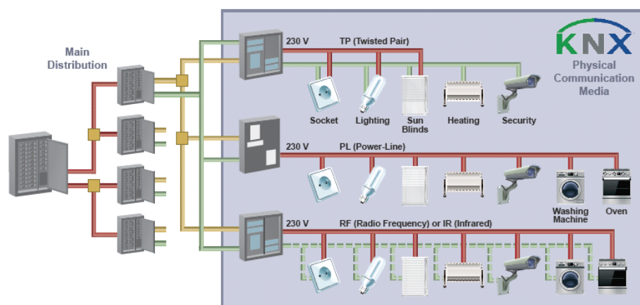
图 2: KNX 网络通信架构
