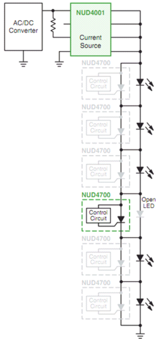
图 4: 用 NUD4700 保护 LED 串
