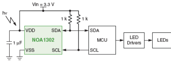
图 3: NOA1302 环境光传感器
