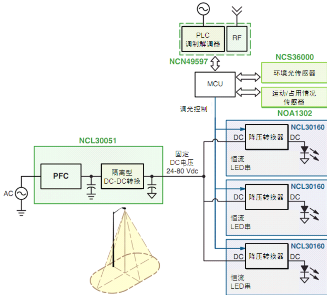
图 1：安森美半导体用于智能 LED 街灯的调制解调器、电源及传感器方案概览
