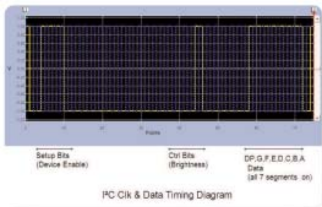
► 图 7. I 2 C 时钟和数据要求。
