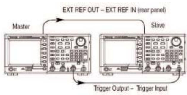
► 图 6. 同步两部 AFG3000 系列仪器。
