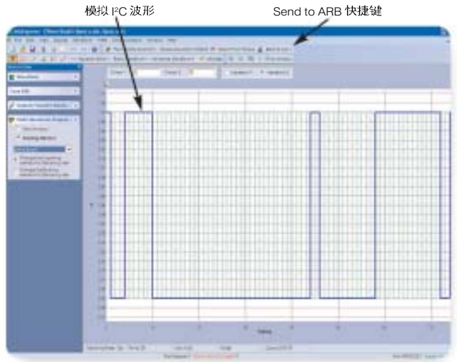
► 图 10. 作为重叠的模拟波形显示的 I 2 C 时钟和数据。
