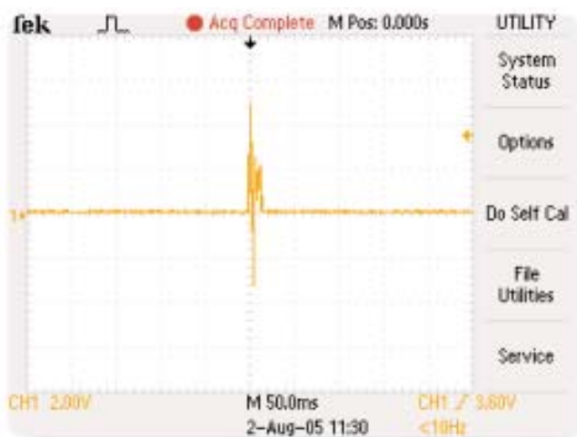
► 图2. 示波器上捕获的爆震传感器。
