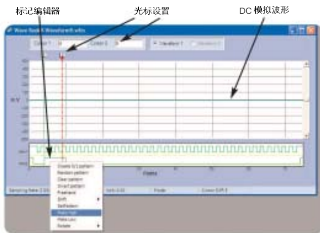
► 图 8. ArbExpress 标尺 "Make High" 功能。
