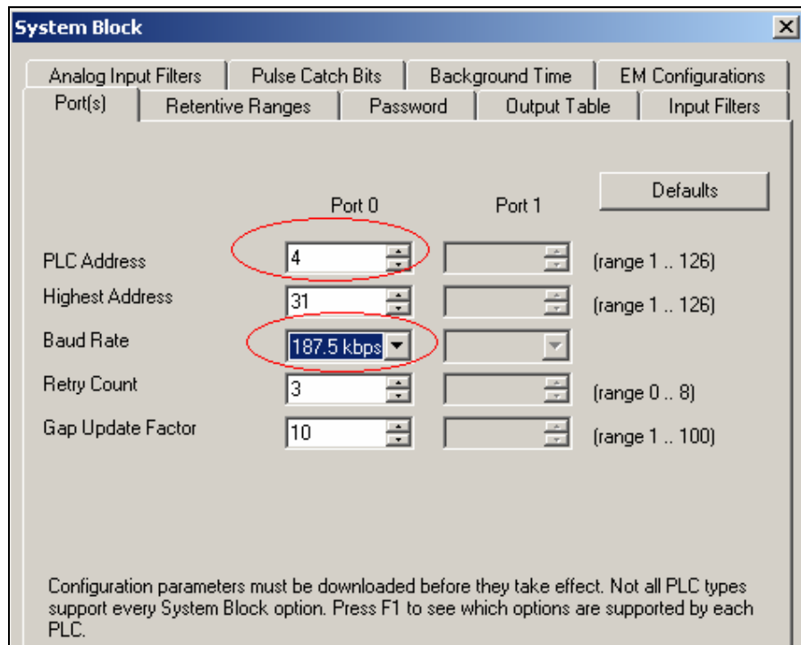
图 3 设置 S7-200 MPI 接口
