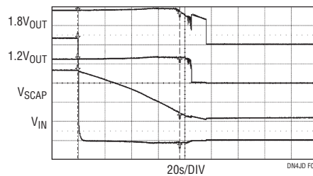
图 2：支持一个 20W 负载的超级电容器备份时间
