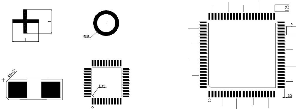
图 23 丝印图形公共要素尺寸要求
