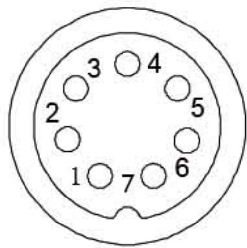
7pin
