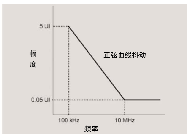
图 7. 正弦曲线抖动压力模板。
