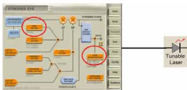
图 6. 直接来自 BERTScope 的正弦曲线干扰源驱动激光器进行光接口接收机测试。
