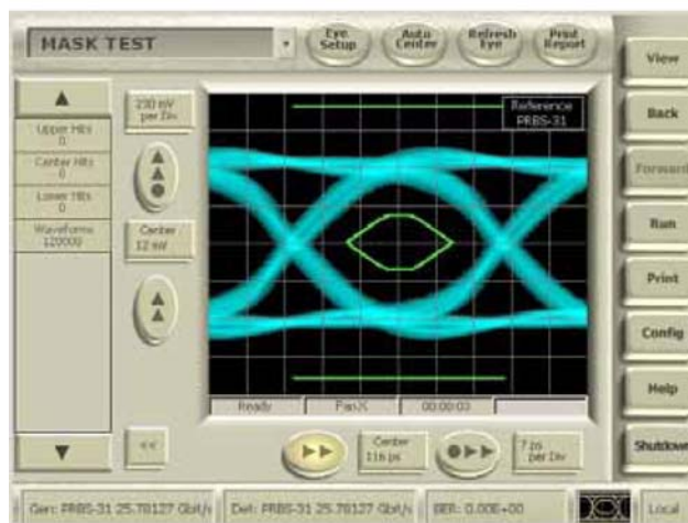
图 4b. BERTScope 上的 100GbE 眼图模板。
