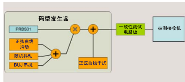
图 14. 加压电接口接收机测试设置。
