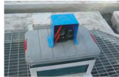
自动加药设备 / Flocculant Add Device
