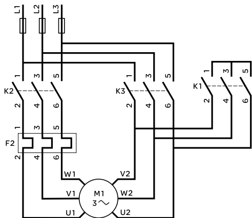
电源图 RE7 YA12BU
