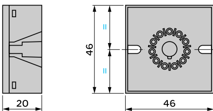
11- 针基座 RE 48A SOC11 AR
