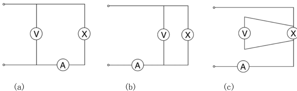
(a) 电流表内接法；(b) 电流表外接法；(c) 四线法电压取样
