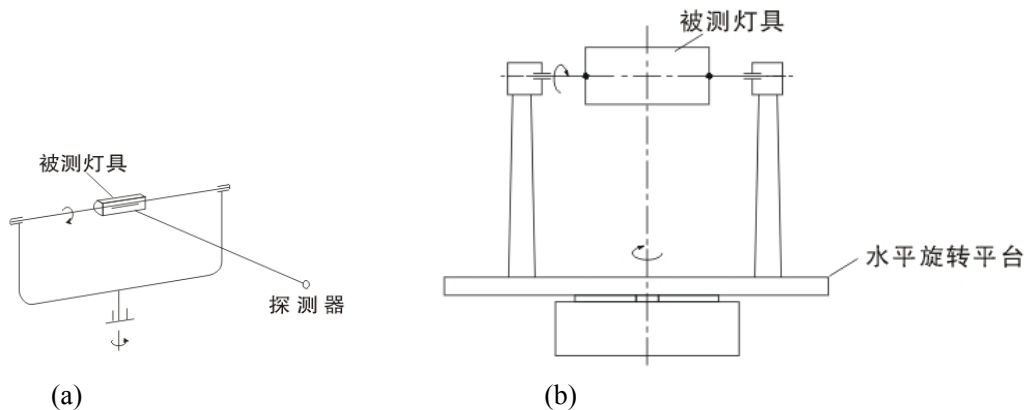
图6 典型灯具旋转式分布光度计原理(a)和转台结构(b)示意图
