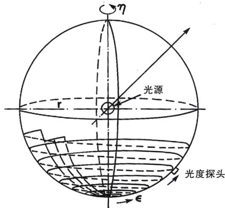
图4 光通量的计算原理示意图
