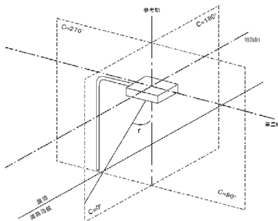
图1 LED 路灯光分布的坐标系统
