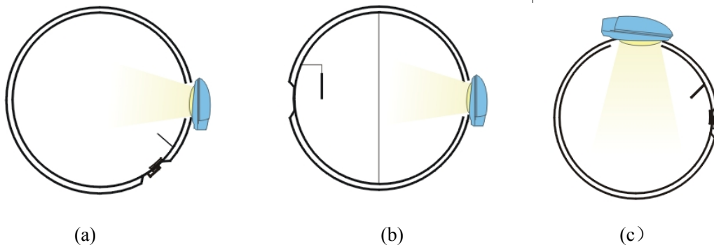
图2 用积分球测量 LED 路灯的示意图
