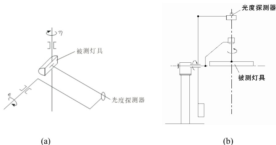
图5 CIE 84 推荐的测量光通量的基准分布光度计原理(a)和结构(b)示意图
