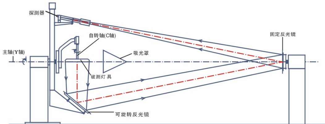
图7 双镜分布光度计示意图
