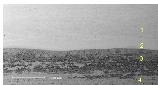
1-熔覆层; 2-结合层; 3-热影响区; 4-基材 (基材: 45 钢)
