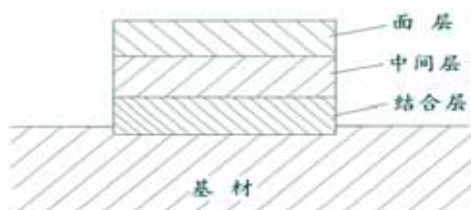
图3 激光熔覆复合层组织示意图
