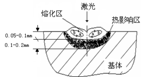
图1 激光熔覆热影响区示意图
