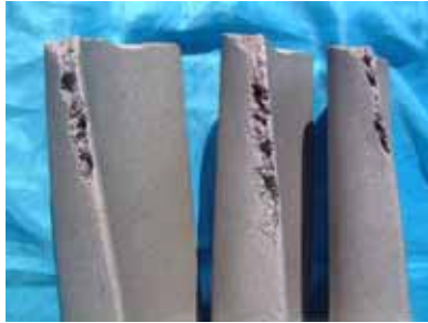
图 4 动叶片损伤状态 Fig.4 Damaged blade
