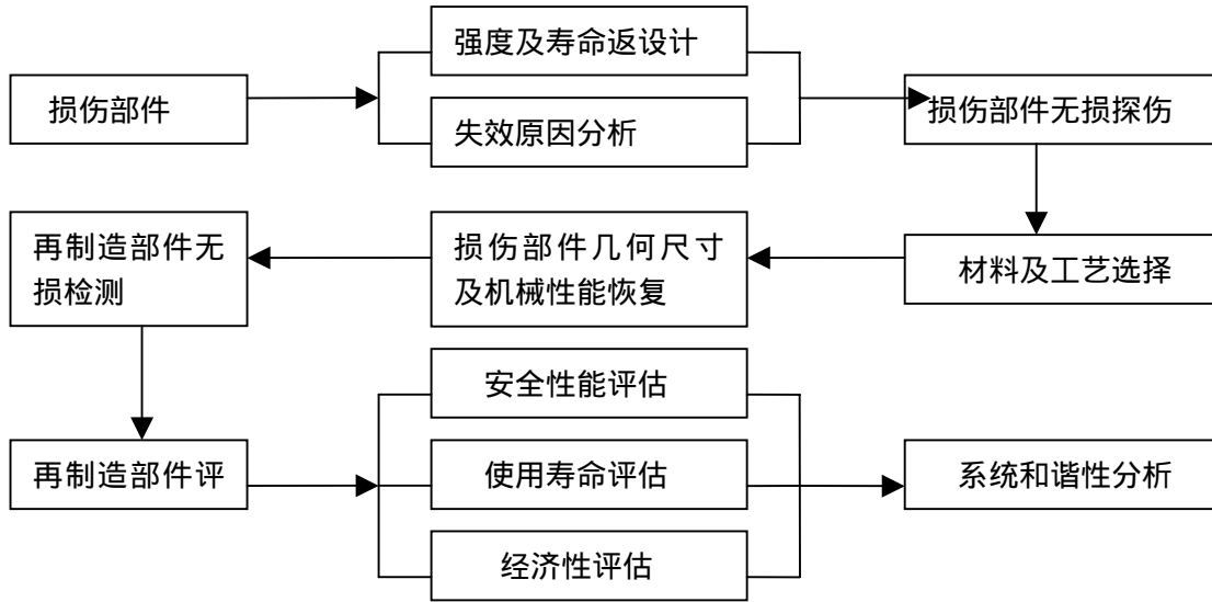
图 15 机械设备激光再制造主要工艺流程图
