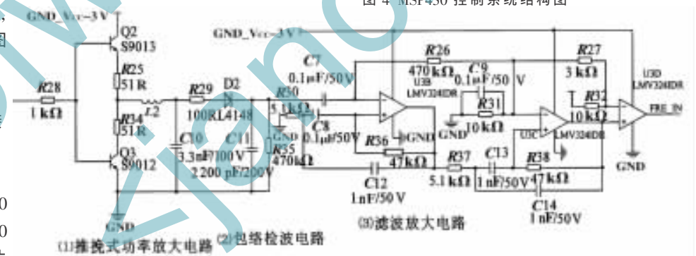
图5 射频卡读写电路
