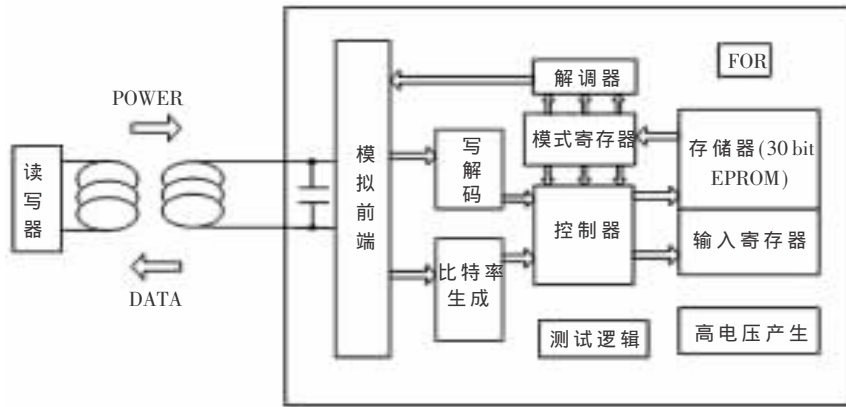
图3 T5557 内部电路组成框图
