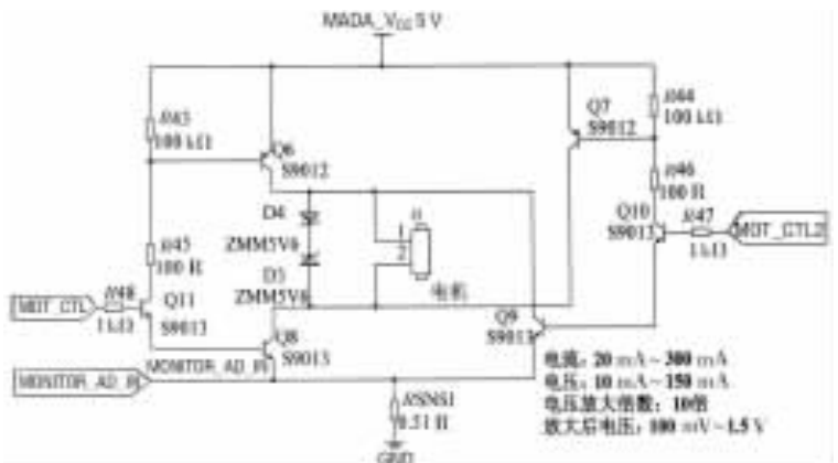
图6 阀门控制电路
