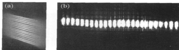
图 10 (a) 阵列近场光斑, (b) 器件微通道单元的典型“smile”
