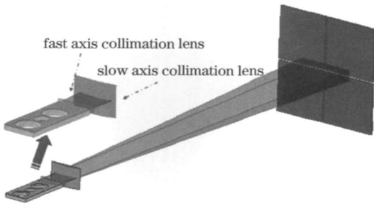
图 2 Bar 条准直及监测装置图
