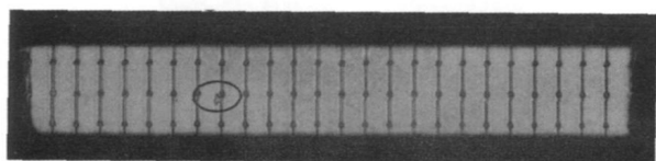
图 8 焊接层内部 SAM 分析
