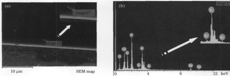
图 4 钎焊料烧焊后激光器腔面扫描电镜图片(a)及元素分析结果(b)
