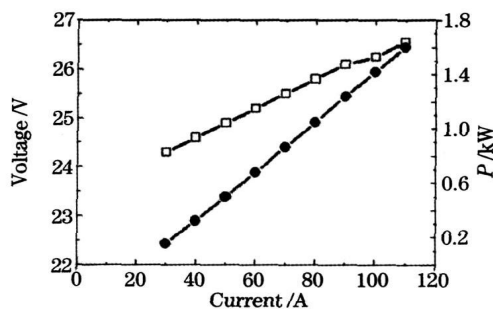
图 11 阵列参数 L-I-V 测试结果
