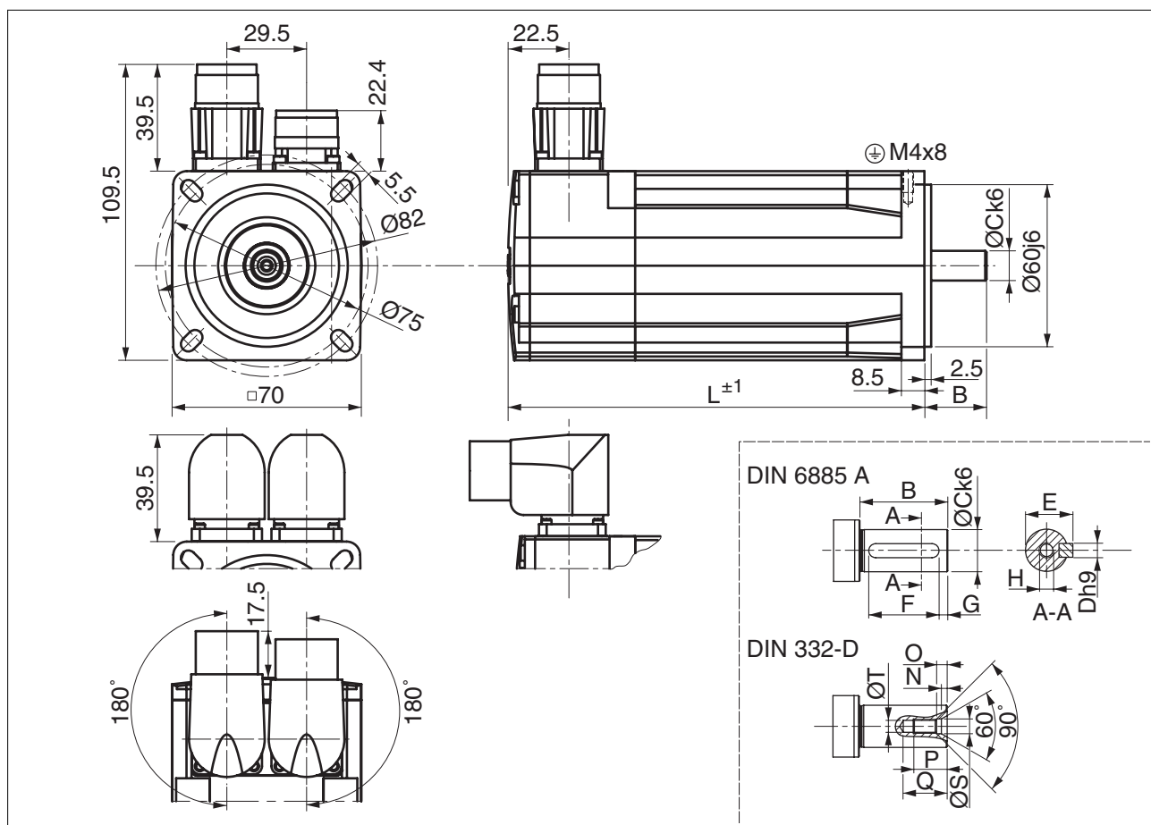
图 2: BMH070 尺寸
