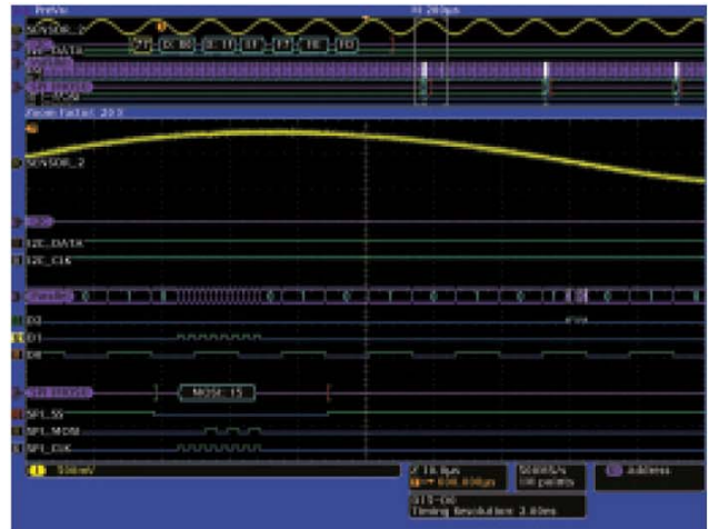
图4. Wave Inspector 用来放大和显示分组细节。
