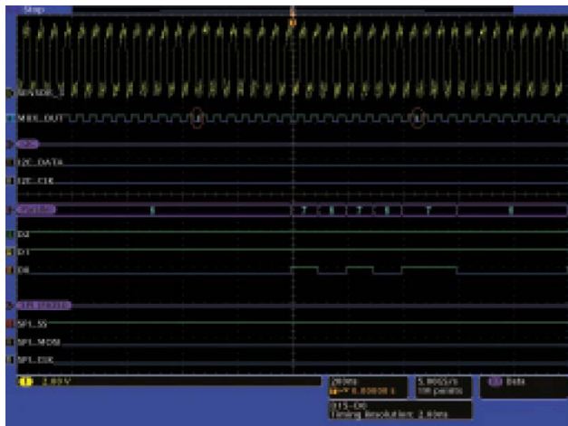
图 5. MUX_OUT 上的白色边沿表明提供了更详细的信息。
