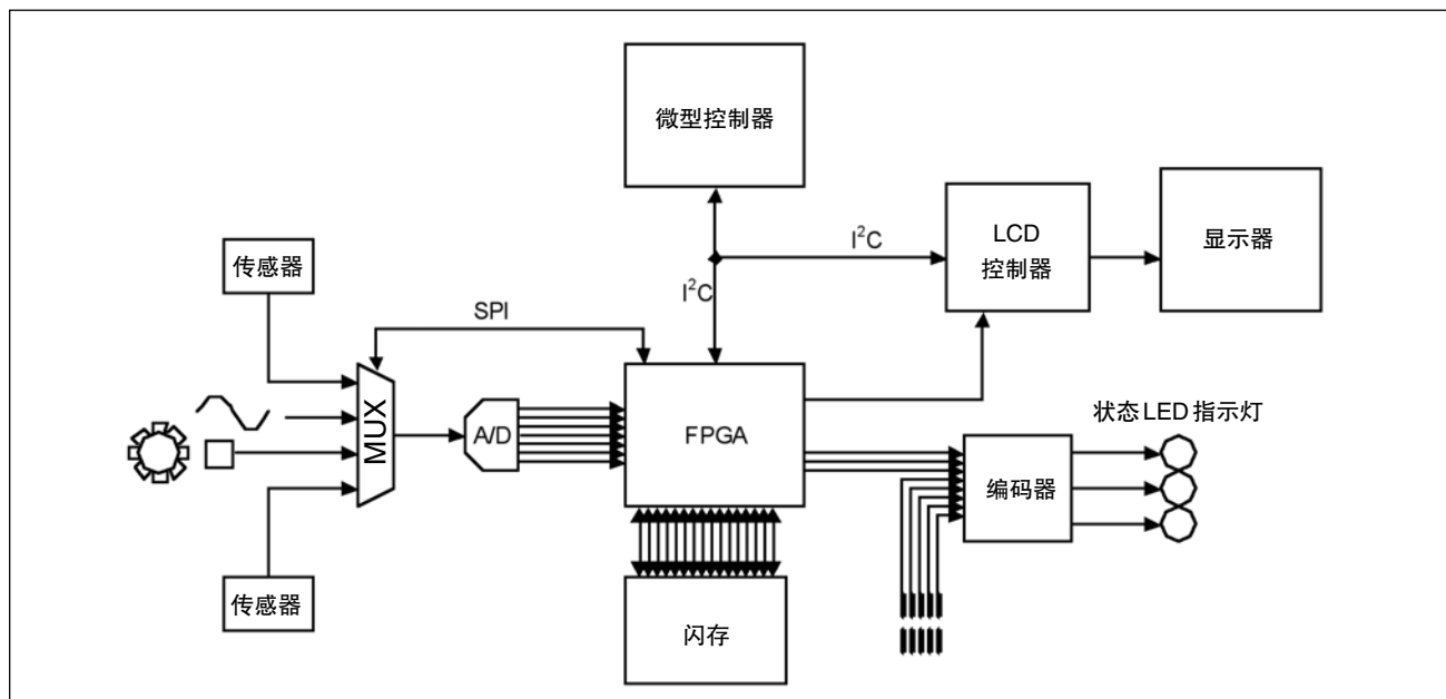
图 1.混合信号嵌入式系统。
