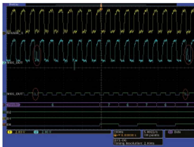
图 7. CH2 显示 MUX_OUT 的更多细节。
