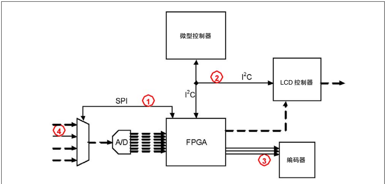
图 2. 带有探测点的采集子系统。
