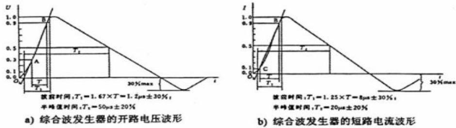
图 8. 试验电压和电流波形
