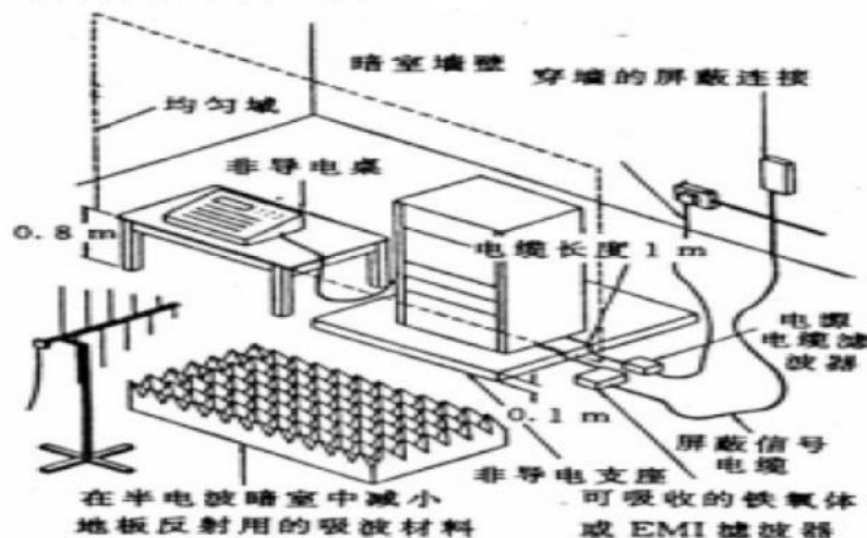
图 6. 射频辐射电磁场抗扰度测试布置图
