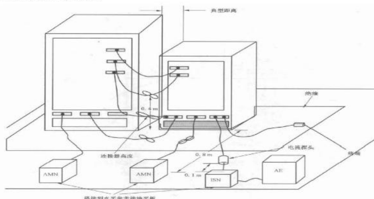
图 3. 传导骚扰测试布置图
