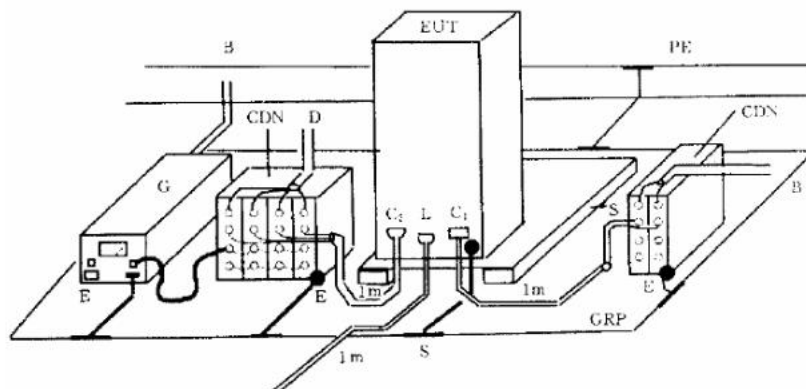
图 11. 阻尼振荡波抗扰度布置图
