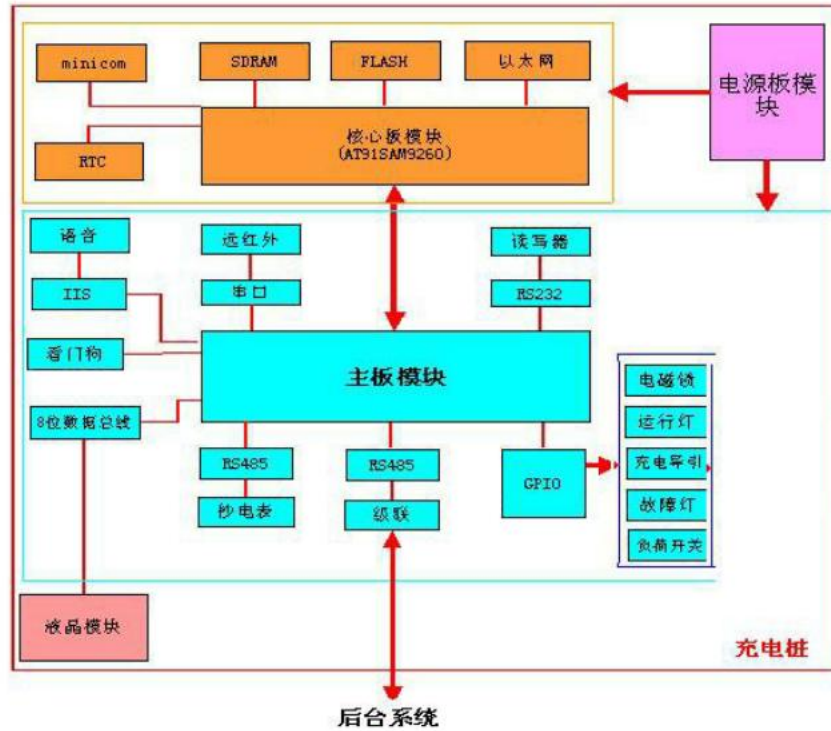
图 1. 交流充电桩的硬件整体框架
