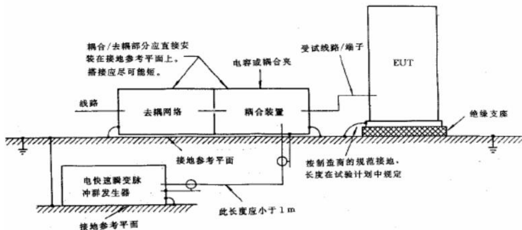
图 7. 电快速瞬变脉冲群抗扰度测试布置图
