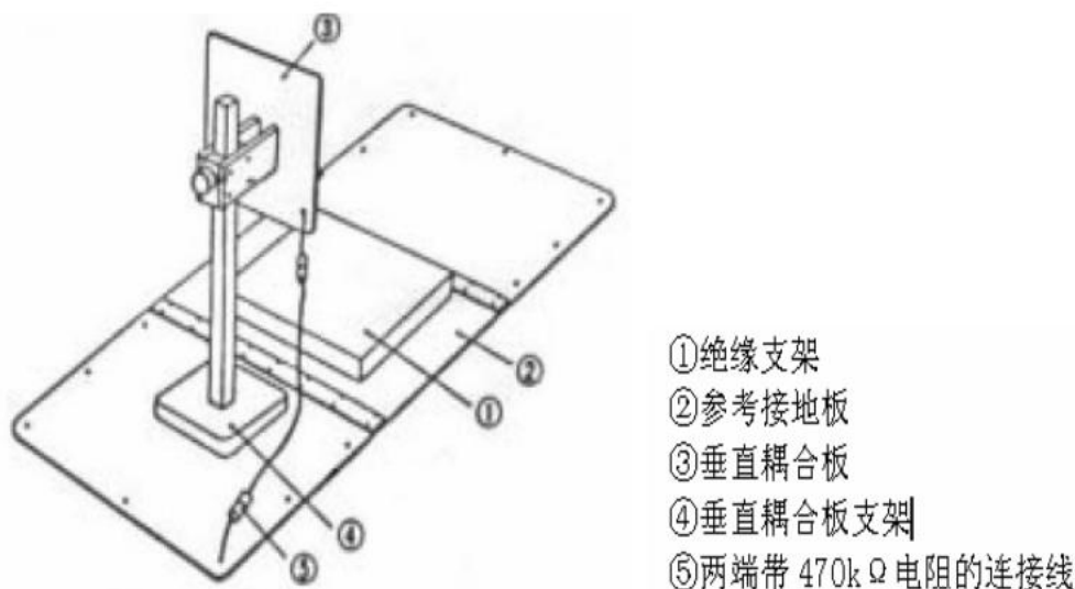
图 5. 静电测试布置图
