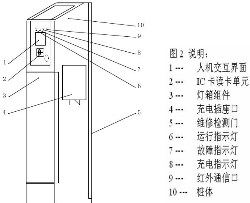
图 2. 交流充电桩的外观示意图
