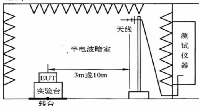
图 4. 辐射发射测试布置图
