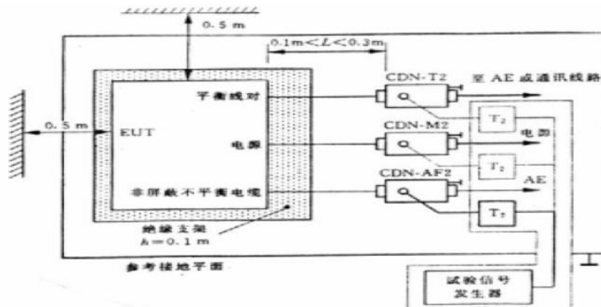
图 9. 射频场感应的传导骚扰抗扰度布置图
