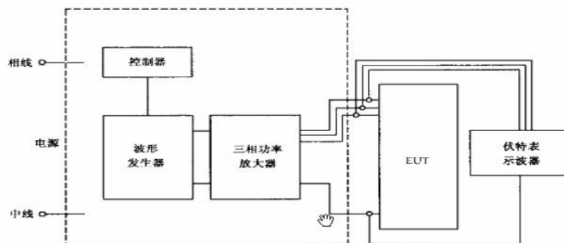
图 10. 电源电压跌落、瞬时中断及电压变化抗扰度布置原理图
