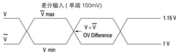
逻辑分析仪查看的等效差分输入 (300mV 摆幅) 和探头模拟输出 **
