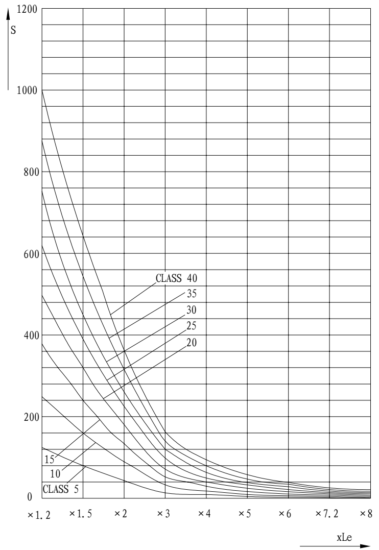
过载特征曲线
