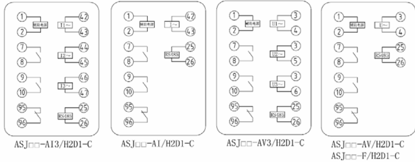
5.3 接线方法（注：如与仪表壳体上接线图不一致，以仪表壳体上为准）□
